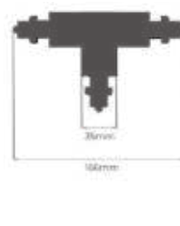
10400 ○ Blanco / White 10401 ● Negro / Black Conector (T) Trifásico Track (T) a join Trifasic
